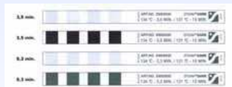
ISP Helix Test System Prodotto conforme alla EN 867-5 Indicatore conforme alla EN ISO 11140-1, Classe 2 + 6
